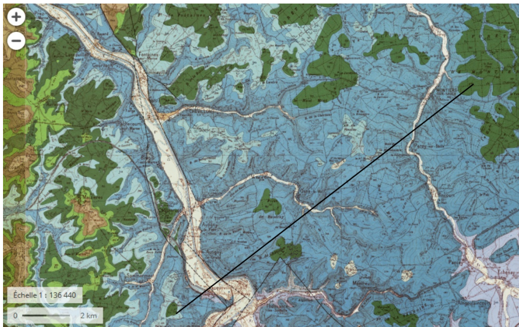
FIGURE 6. EXTRAIT DE LA CARTE GEOLOGIQUE DE JOINVILLE (ISSUE DE GEOPORTAIL), AVEC POSITION DU TRAIT DE COUPE (TRAIT NOIR EPAIS NE-SW)
